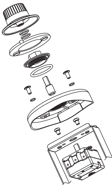
Carcasa con perilla de termostato externa con IP69K de protección contra el ingreso
