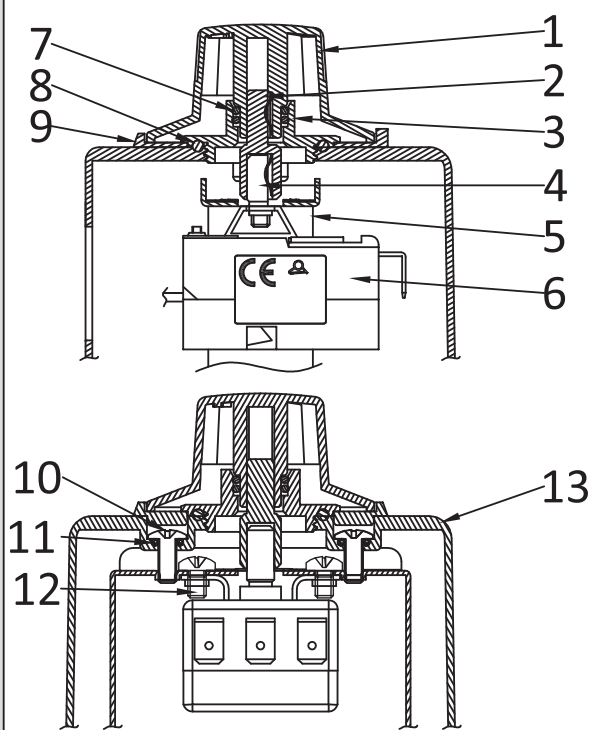
Carcasa con perilla de termostato externa con IP69K de protección contra el ingreso
