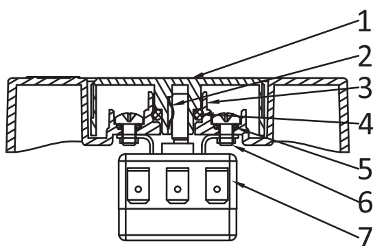
Carcasa con perilla de termostato externa con IP69K de protección contra el ingreso
