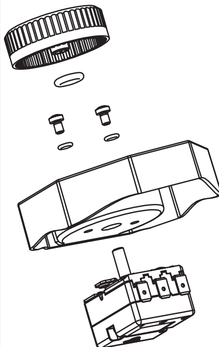
Carcasa con perilla de termostato externa con IP69K de protección contra el ingreso
